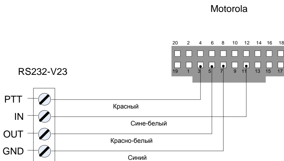
Рисунок 6 Подсоединение к радиостанции
