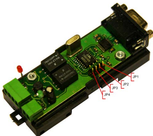
Рисунок 5 Соответствие контактов разъема обозначениям перемычек
