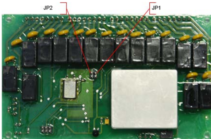
Рисунок 6 Вид платы, технологические переключки
