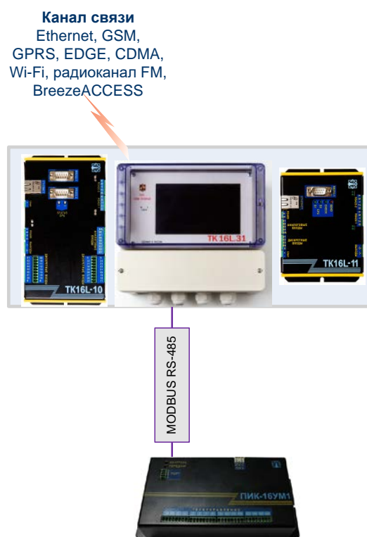
Рисунок 4 Архитектура системы, нижний уровень
