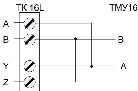
Рисунок 5 Схема подключения к RS-422
