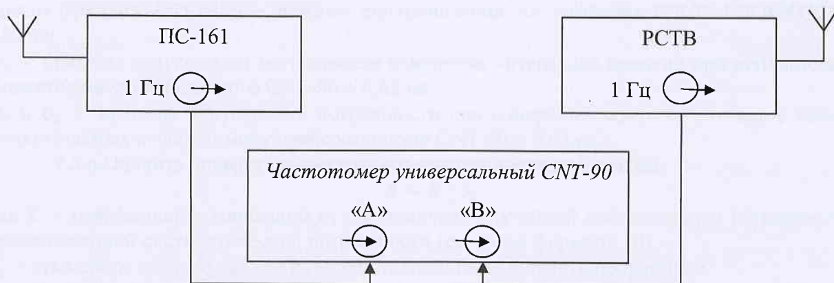
Рисунок 1 – Схема определения смещения формируемой ШВ относительно национальной ШВ UTC(SU) в режиме синхронизации по сигналам ГНСС ГЛОНАСС/GPS
