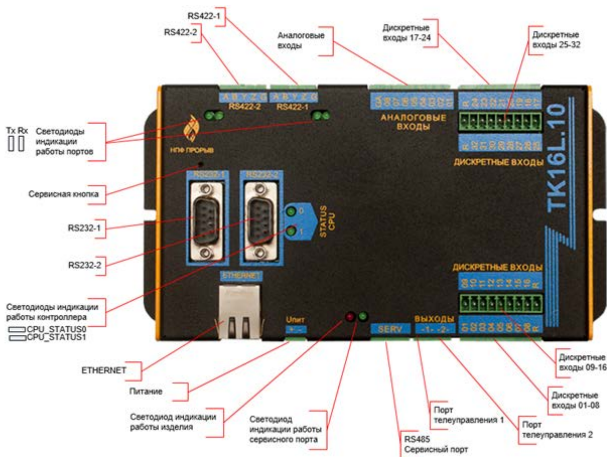
Рисунок 3 Вид панели аппаратного блока с элементами подключения и индикации
