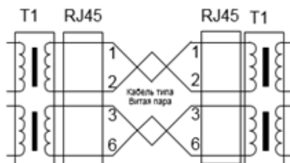
Рисунок 8 Схема подключения к HUB
