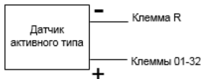
Рисунок 11 Подключение датчика активного типа
