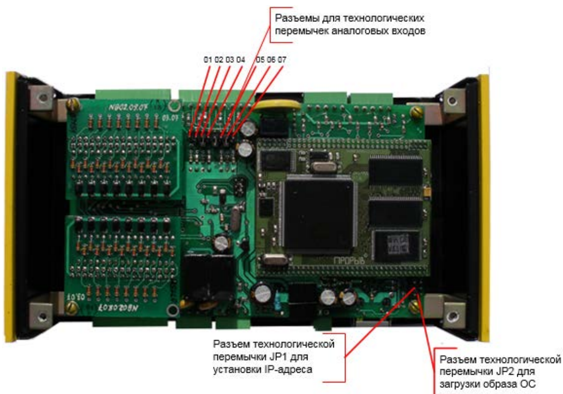
Рисунок 12 Вид платы, технологические перемычки
