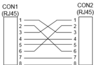
Рисунок 9 Схема прямого подключения изделия к компьютеру
