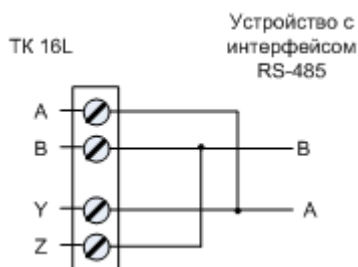
Рисунок 8 Схема подключения RS-485
