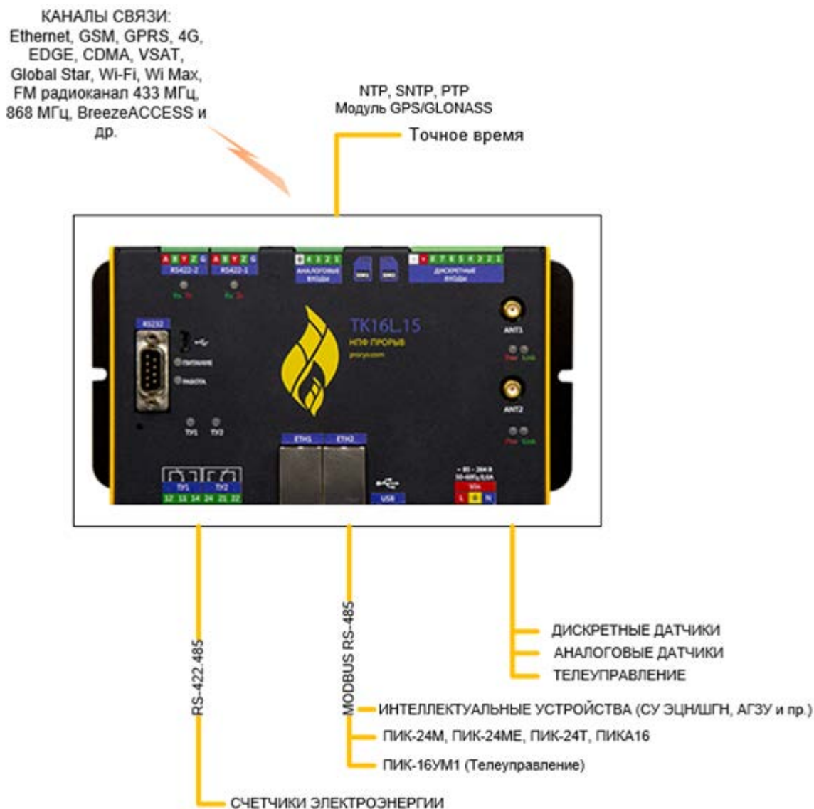
Рисунок 6 Архитектура системы, нижний уровень
