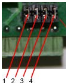
Рисунок 13 Фрагмент платы, разъемы для технологических перемычек
