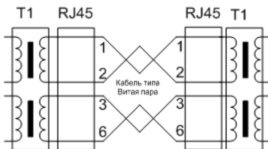
Рисунок 9 Схема подключения к HUB
