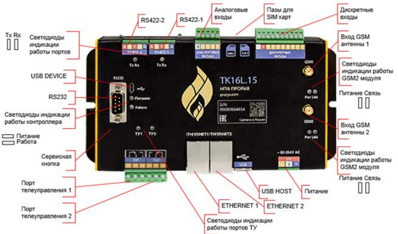
Рисунок 5 Вид панели аппаратного блока с элементами подключения и индикации
