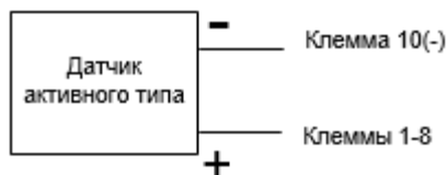
Рисунок 12 Подключение датчика активного типа
