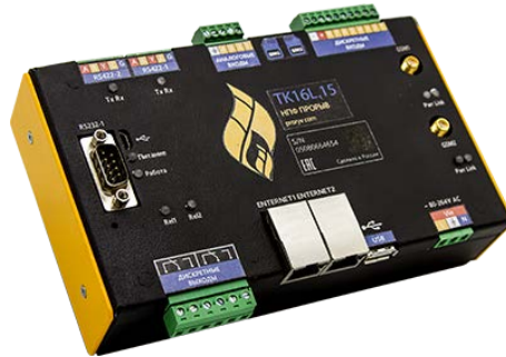
Рисунок 3 Общий вид аппаратного блока изделия в исполнении “Металлический корпус”
