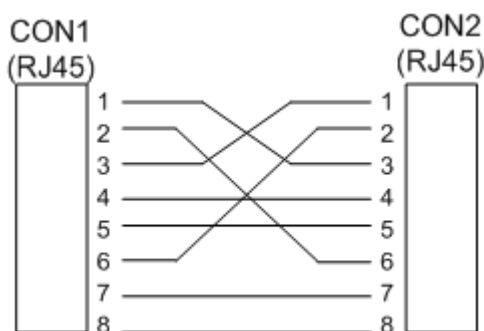
Рисунок 10 Схема прямого подключения изделия к компьютеру
