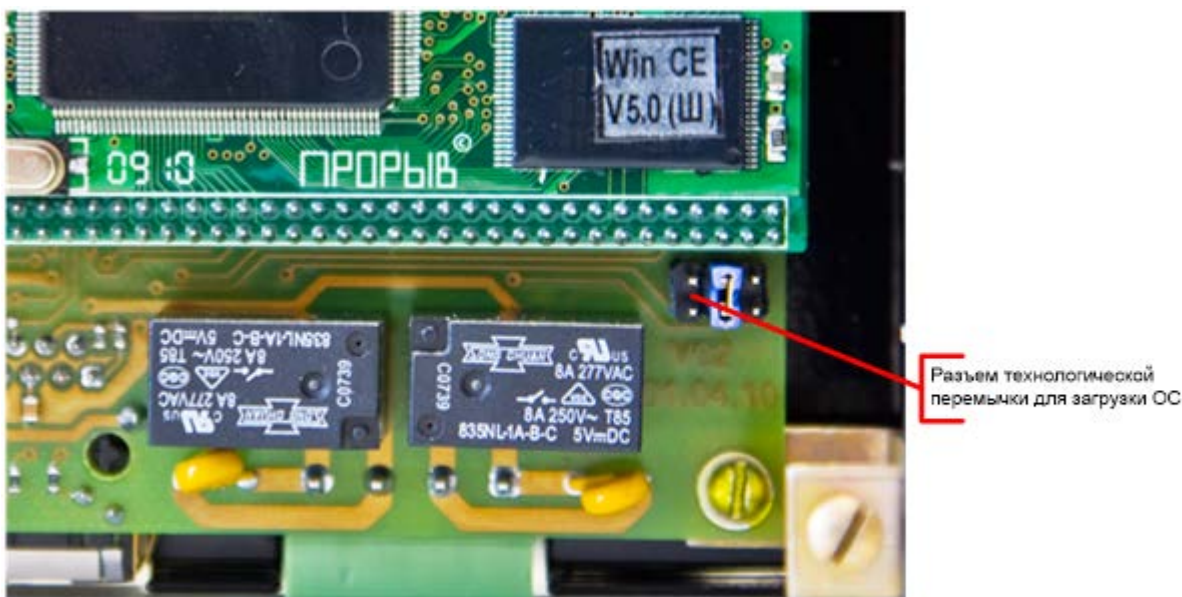
Рисунок 16 Положение технологической перемычки JP2
