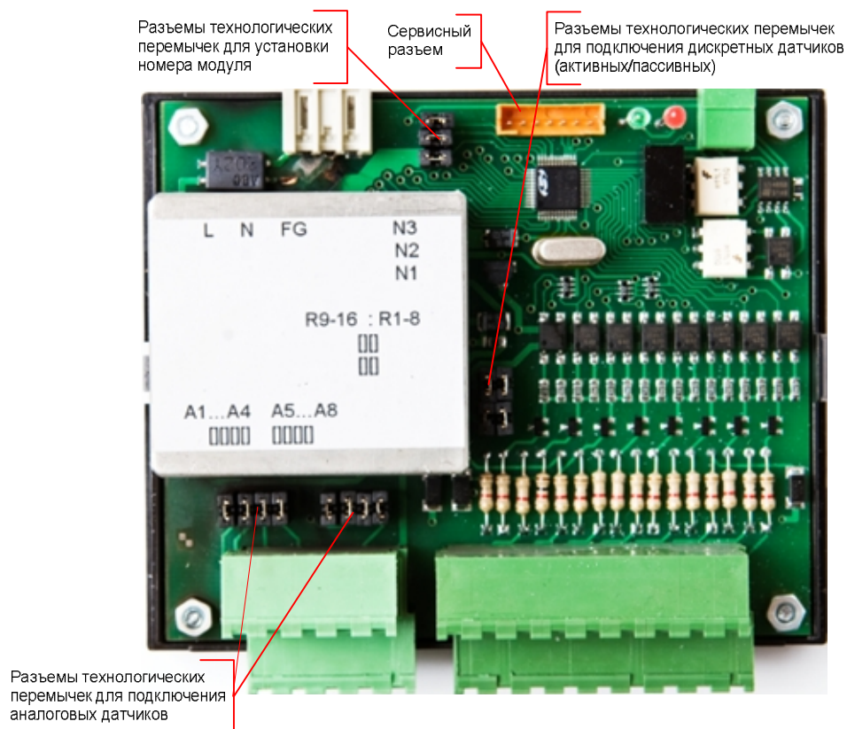
Рисунок 6 Вид платы, технологические перемычки
