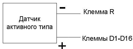
Рисунок 10 Подключение датчика активного типа
