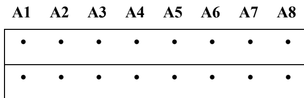
Рисунок 13 Соответствие контактов разъема А1...А4 А5...А8 входным каналам
