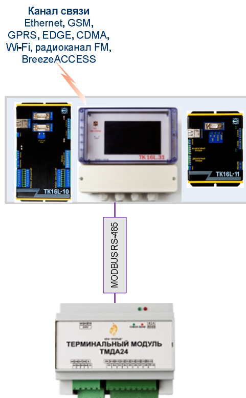
Рисунок 4 Архитектура системы, нижний уровень
