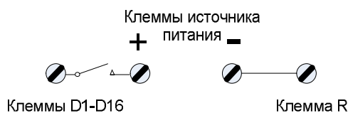
Рисунок 7 Подключение датчика ТС типа “сухой контакт”
