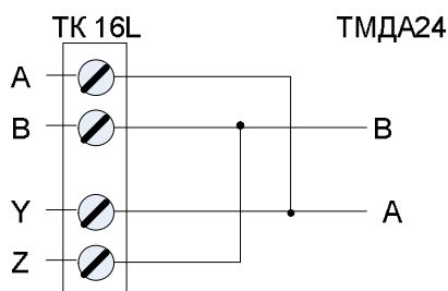
Рисунок 5 Схема подключения к RS-422
