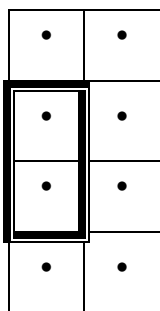
Рисунок 12 Установка технологических перемычек для подключения активных датчиков (D9-D16)
