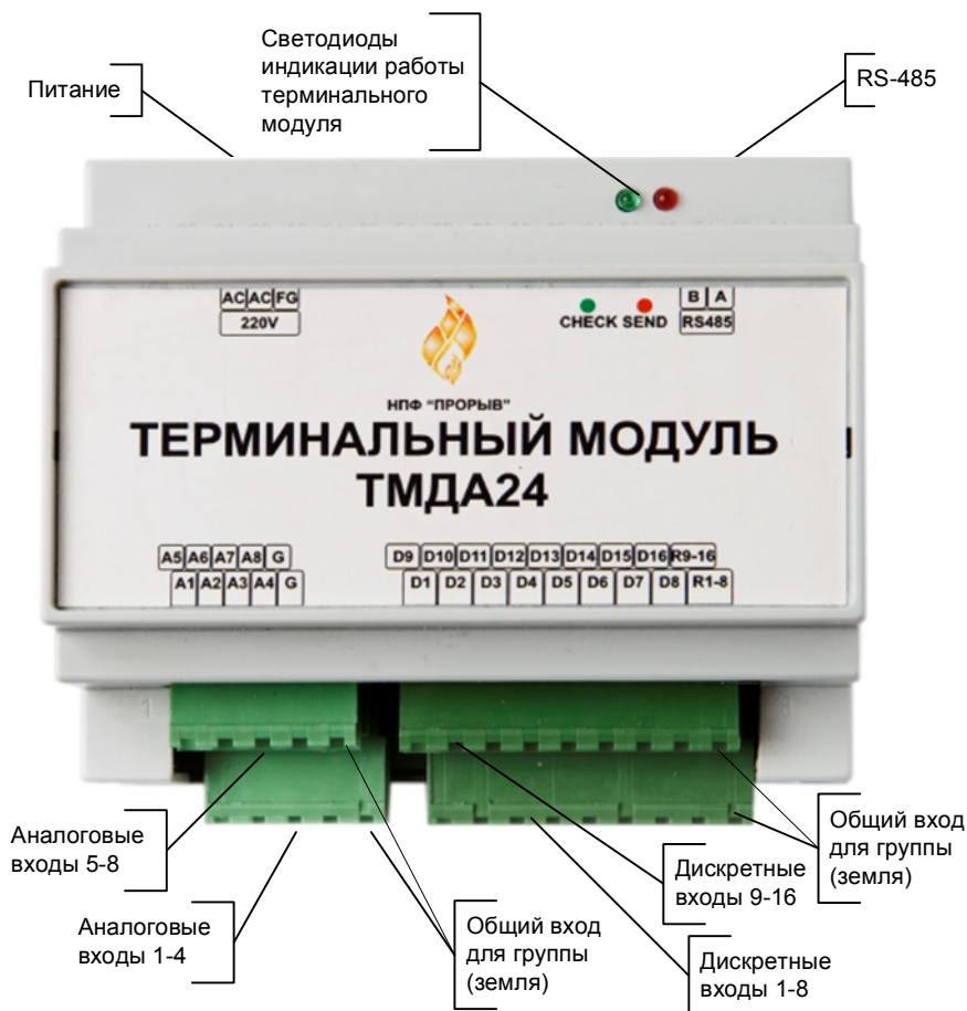
Рисунок 3 Вид панели аппаратного блока с элементами подключения и индикации
